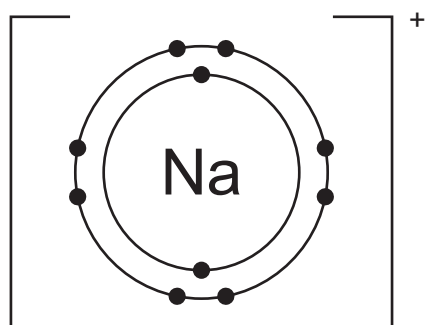
sodium ion
