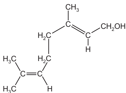
geraniol
